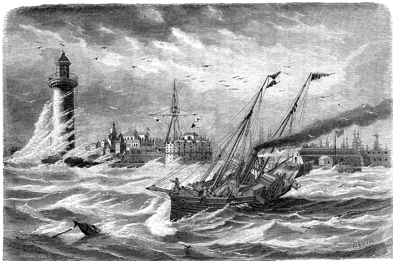
Sl. 38. Jaka plima (za ekvinokcija ili jednači dana i noći) u Havru.
