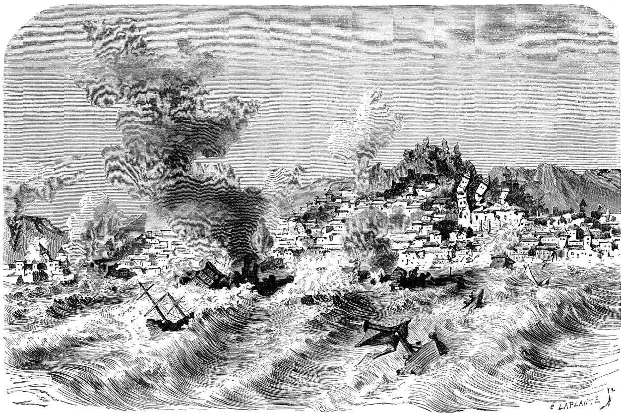
Sl. 12. Lizabonski potres 1. studenoga 1755.
