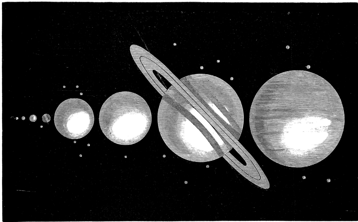
Sl. 2. Razmjerna veličina obhodnica (planeta). 1. Merkur; 2. Mart; 3. Venera; 4. Zemlja; 5. Uran; 6. Neptun; 7. Saturn sa prstenom; 8. Jupiter.
