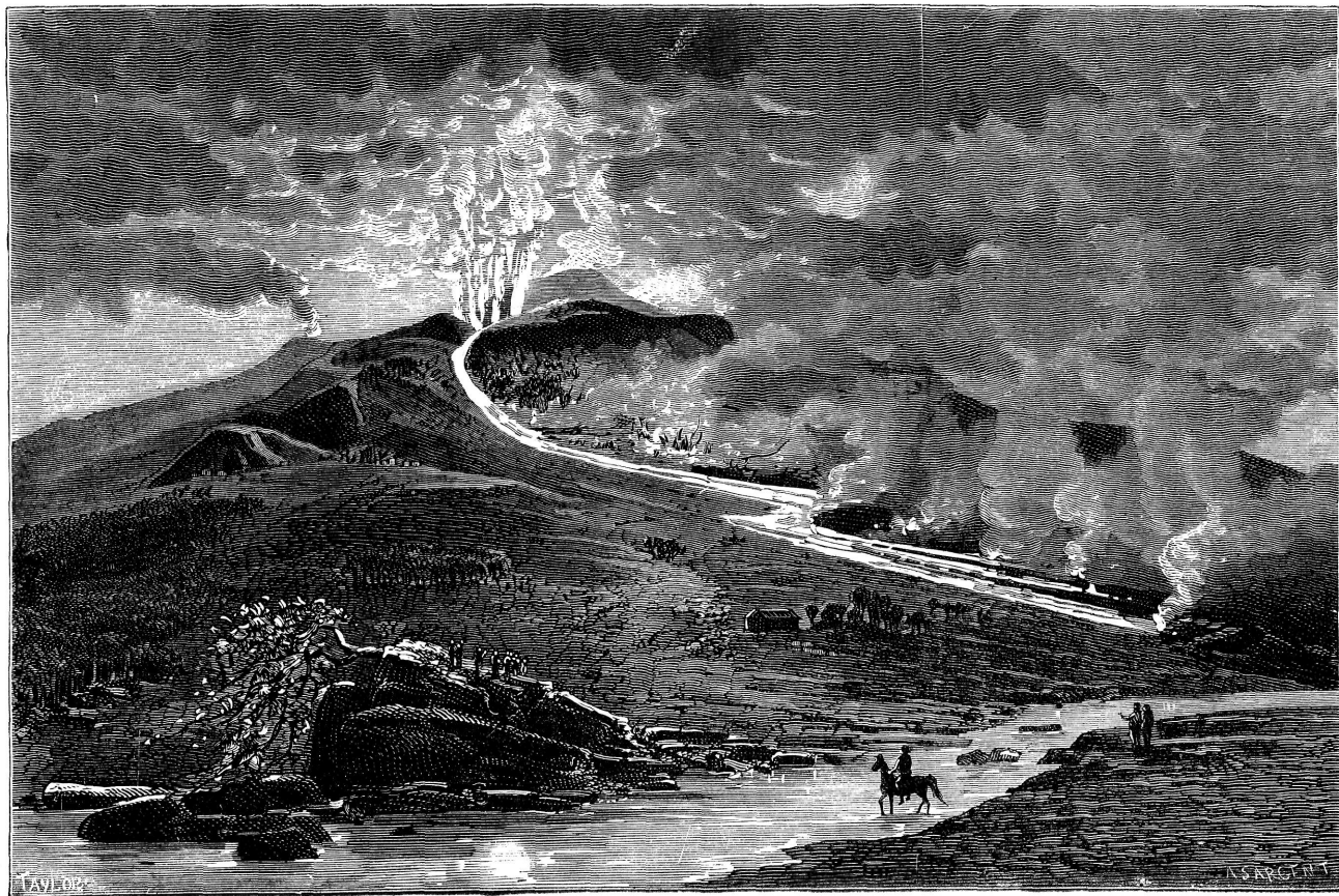
Sl. 9. Provala Etne g. 1879.
