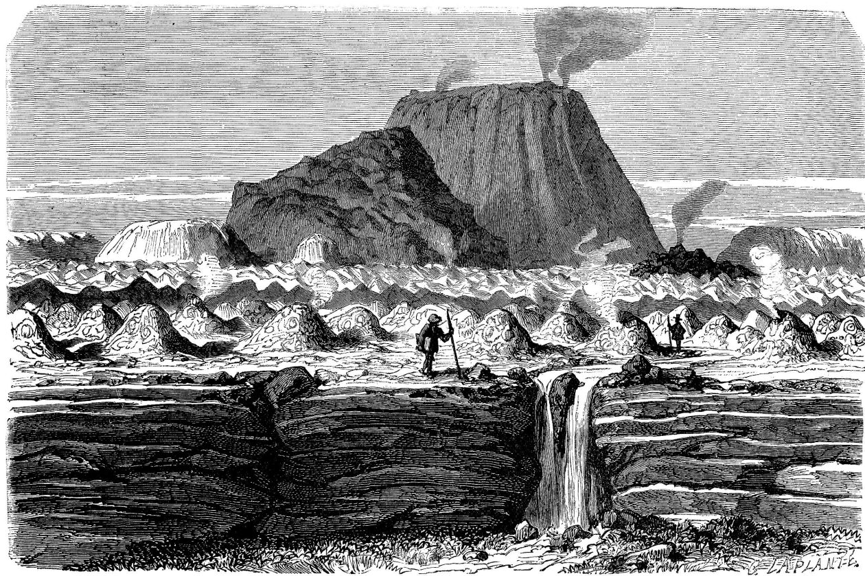
Sl. 8. Vulkan Jorullo u Meksiku.
